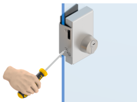
Instalación en puerta Mod. EP15 y EP15-H
