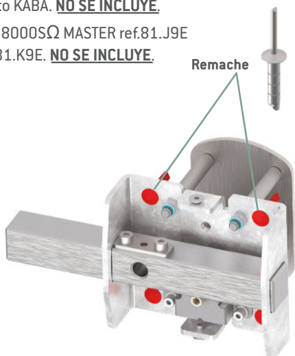
GRAMPÓN Tipo A (Para puerta sin solape)
