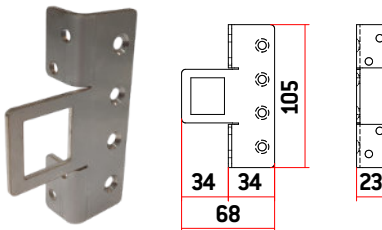
Grampón tipo A
